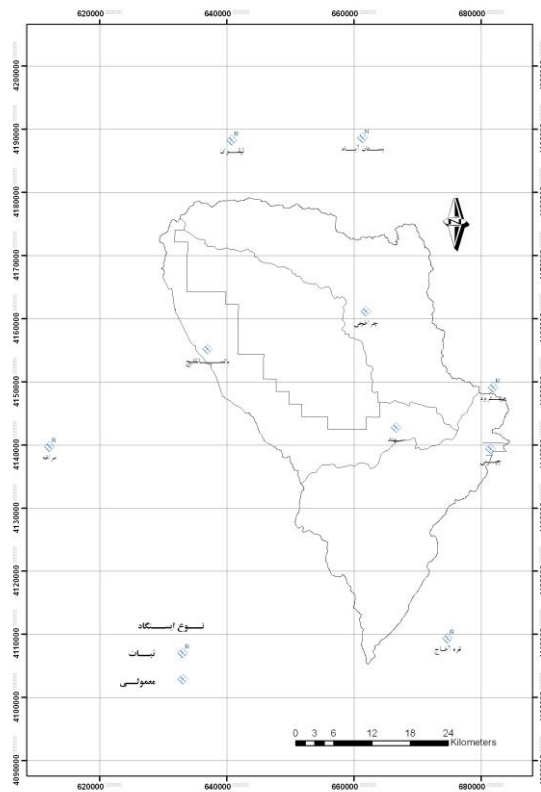
شکل ۳. موقعیت ایستگاه‌های باران‌نگار و باران‌سنج واقع در محدوده مورد مطالعه
