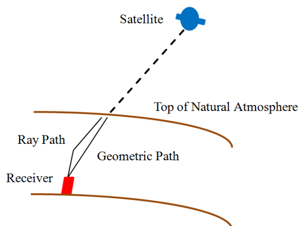
شکل ۱: شکست مسیر موج ارسالی به دلیل عبور از لایه‌هایی با ضریب شکست متفاوت [۶]
