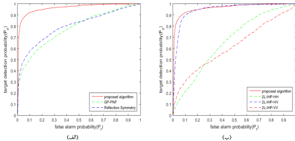
شکل ۹: منحنی ROC مربوط به (الف) روش پیشنهادی و GP-PNF و تقارن بازتابی، (ب) روش پیشنهادی و 2L-IHP در کانال‌های HH و HV و VV
