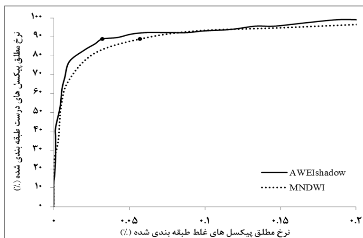
شکل ۸: صحت طبقه‌بندی پیکسل‌های مربوط به پیکسل‌های آب خالص رودخانه برای آستانه‌های مختلف با استفاده از نمودار ROC
