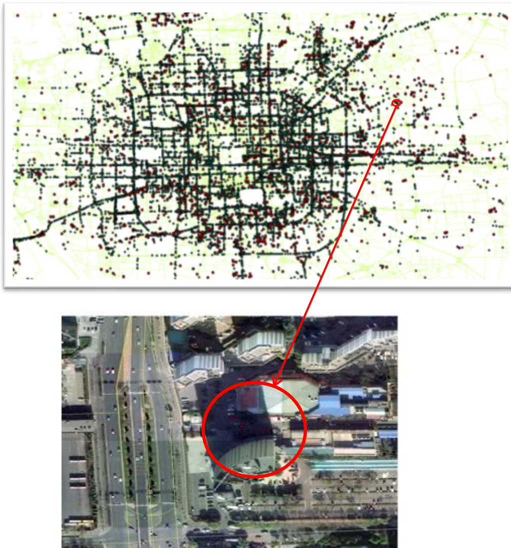
شکل ۲: خوشه‌بندی مکانی زمانی DBSCAN بر روی کل شبکه شهر پکن و بزرگنمایی یکی از مناطق شناسایی شده جهت حذف پارکینگ
