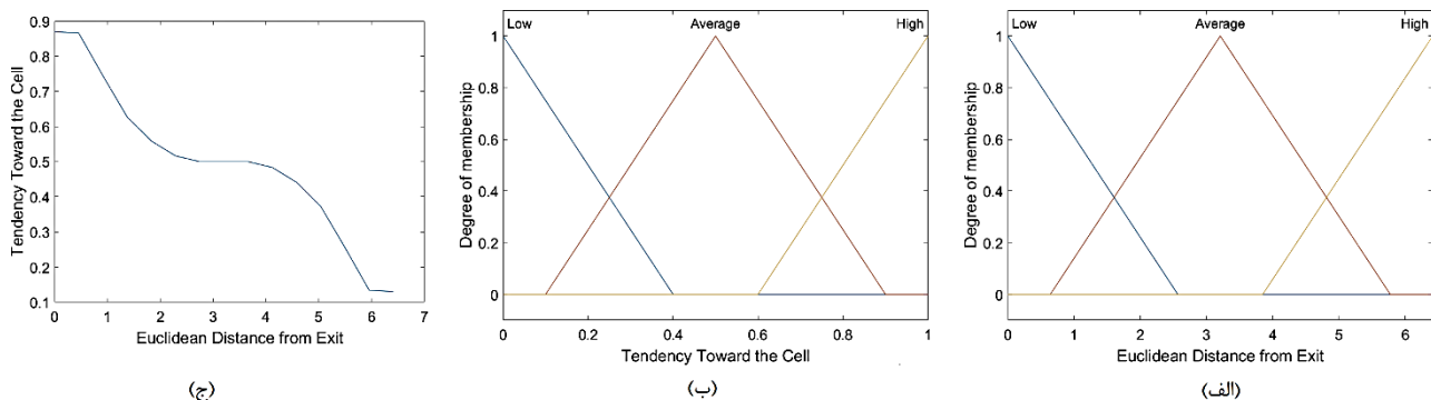
شکل ۴: نمایش سیستم فازی برای فاصله از خروجی. (الف) تابع عضویت برای فاصله از خروجی، (ب) تابع عضویت فازی برای میزان تمایل به رفتن به سلول، (ج) نتیجه‌ی سیستم فازی بر اساس قوانین ذکر شده
