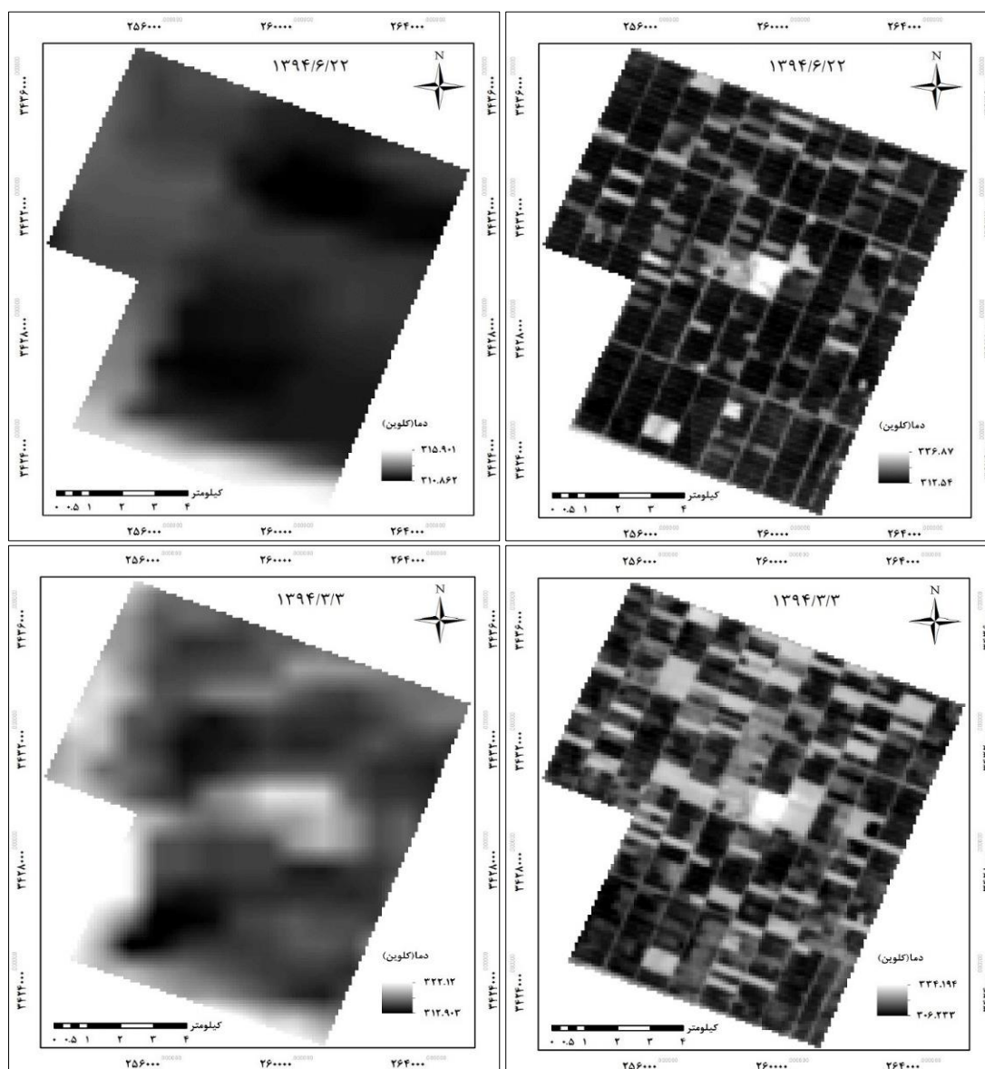
شکل ۳: تصاویر ورودی لندست و مادیس تاریخ‌های ۳ خرداد و ۲۲ شهریور (کلوین).
