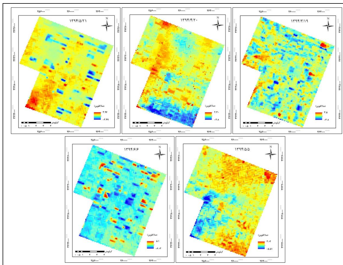
شکل ۷: اختلاف دمای سطح پیش‌بینی شده و دمای سطح مشاهده شده برای تاریخ‌های مختلف (کلون)
