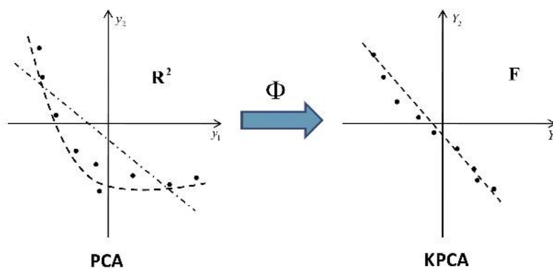
شکل ۲: ایده اصلی استفاده از KPCA با هسته کرنل غیرخطی [۲۳]
