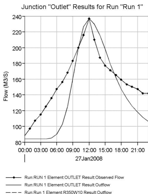
شکل ۸. مقایسه هیدروگراف مشاهده‌ای و شبیه‌سازی در مرحله واسنجی حوضه قرنقو در تاریخ ۸۴/۱/۲۷
