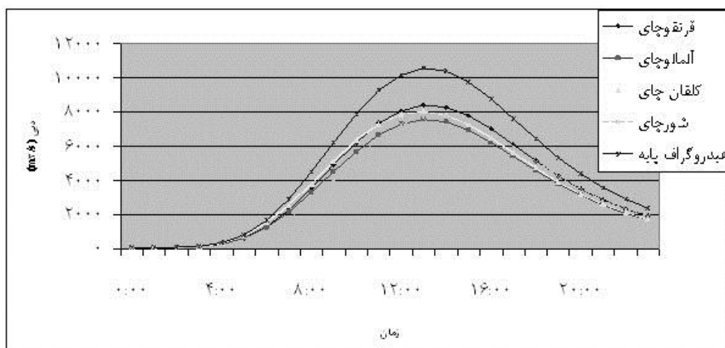
شکل ۹. مقایسه هیدروگراف خروجی حوضه پس از حذف هیدروگراف زیرحوضه‌ها برای بارش طراحی
