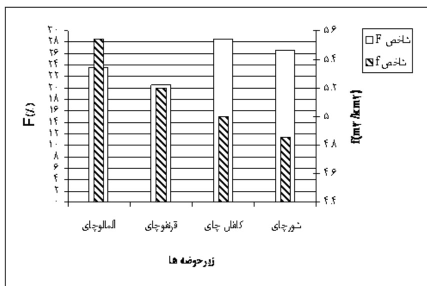
شکل ۱۰. نمودار مقایسه‌ای شاخص‌های F و f زیرحوضه‌های حوضه آبخیز قرنقو
