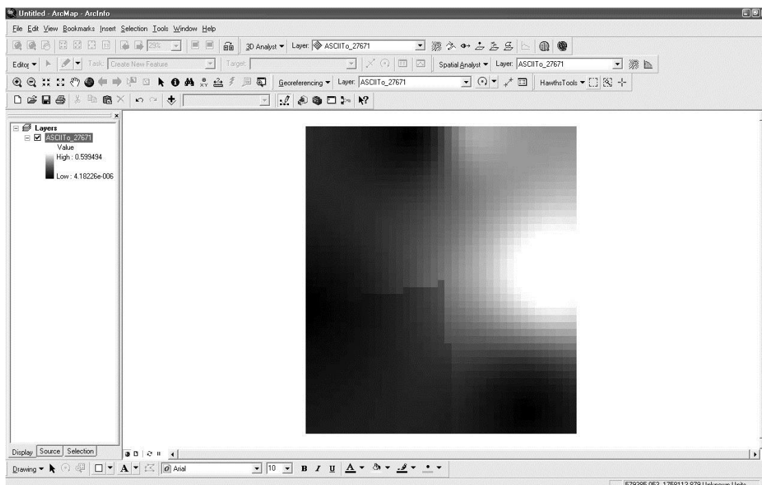
شکل ۷. نمونه‌ای از شبکه بارش با اندازه سلول 2 \times 2 کیلومتر در محیط GIS
