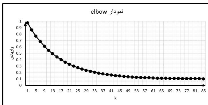
شکل ۴: نمودار elbow برای داده های مورد مطالعه
