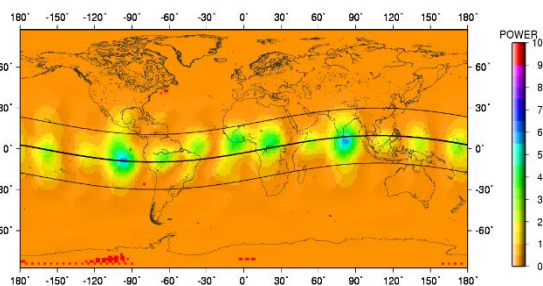
شکل ۱: مقدار توان طیفی پریود یک پنجم روزانه با ضریب 10^{-4} شکل ۲: مقدار توان طیفی پریود یک چهارم روزانه با ضریب 10^{-4}
