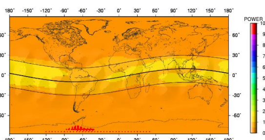
شکل ۵: مقدار توان طیفی پریود روزانه با ضریب 10^{-7} شکل ۶: مقدار توان طیفی پریود ۲۷ روزه با ضریب 10^{-3}
