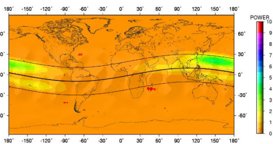
شکل ۷: مقدار توان طیفی پریود \frac{1}{4} سالانه با ضریب 10^{-4} شکل ۸: مقدار توان طیفی پریود \frac{1}{3} سالانه با ضریب 10^{-5}
