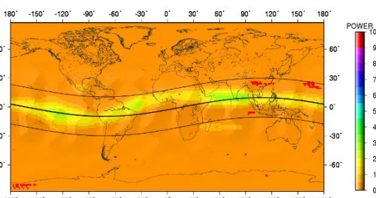
شکل ۳: مقدار توان طیفی پریود یک سوم روزانه با ضریب 10^{-5} شکل ۴: مقدار توان طیفی پریود یک دوم روزانه با ضریب 10^{-5}
