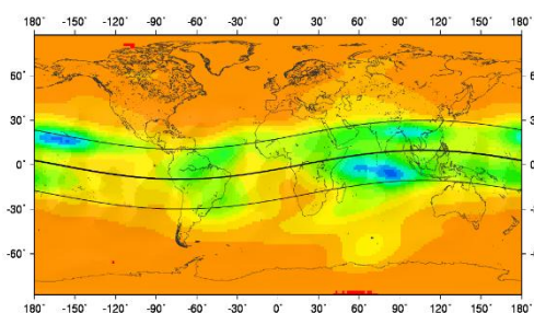
شکل ۳: مقدار توان طیفی پریود یک سوم روزانه با ضریب 10^{-5} شکل ۴: مقدار توان طیفی پریود یک دوم روزانه با ضریب 10^{-5}
