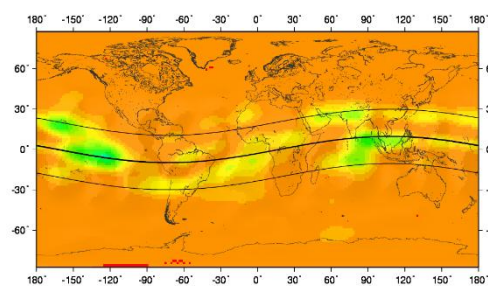
شکل ۱: مقدار توان طیفی پریود یک پنجم روزانه با ضریب 10^{-4} شکل ۲: مقدار توان طیفی پریود یک چهارم روزانه با ضریب 10^{-4}
