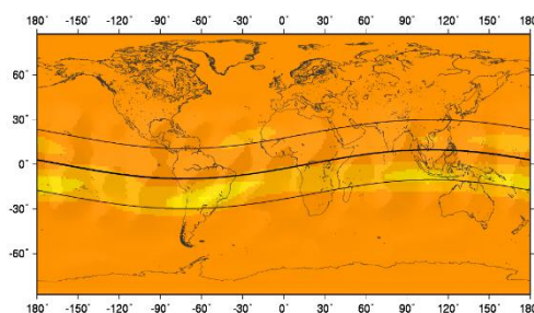
شکل ۷: مقدار توان طیفی پریود \frac{1}{4} سالانه با ضریب 10^{-4} شکل ۸: مقدار توان طیفی پریود \frac{1}{3} سالانه با ضریب 10^{-5}
