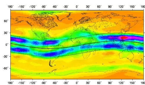
شکل ۵: مقدار توان طیفی پریود روزانه با ضریب 10^{-7} شکل ۶: مقدار توان طیفی پریود ۲۷ روزه با ضریب 10^{-3}
