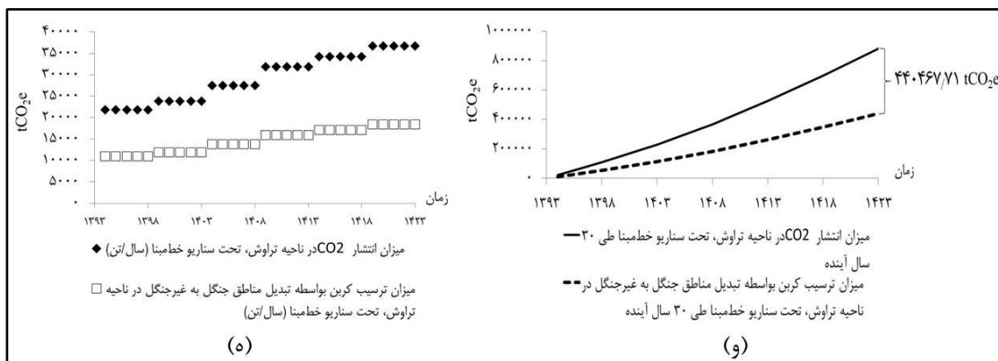
شکل ۱۲: میزان انتشار CO 2 و ترسیب کربن در ناحیه تراوش تحت سناریو خط‌مبنا، (و) نمودار تجمعی میزان انتشار CO 2 و ترسیب کربن در ناحیه تراوش تحت سناریو خط‌مبنا (طی ۳۰ سال آینده)
