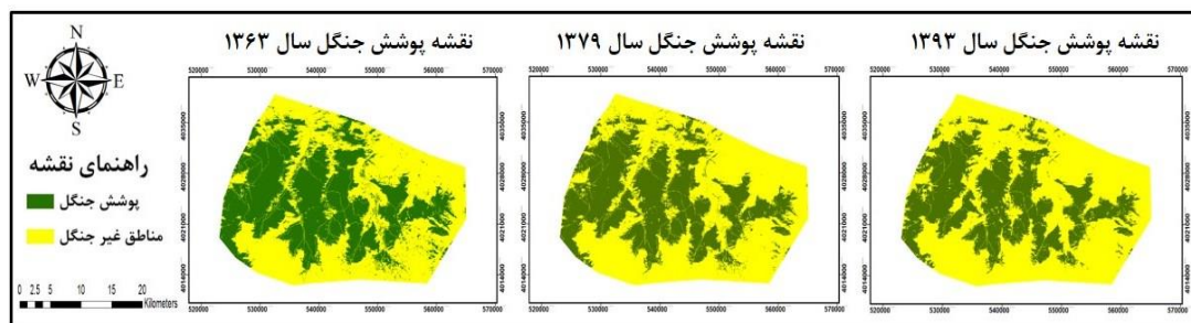
شکل ۵: نقشه های پوشش جنگل منطقه مورد مطالعه
