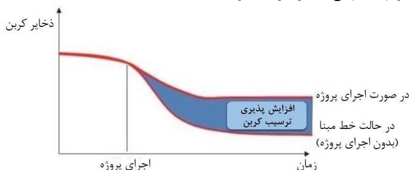
شکل ۱: میزان منابع کربن به واسطه اجرای پروژه REDD [۲۱]
