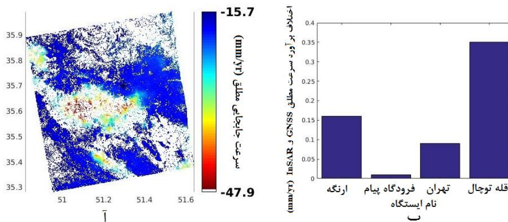
شکل ۱۲: آ- میدان سرعت مطلق و ب- اختلاف برآوردهای سرعت GNSS و InSAR نسبت به هر چهار ایستگاه ژئودینامیک
