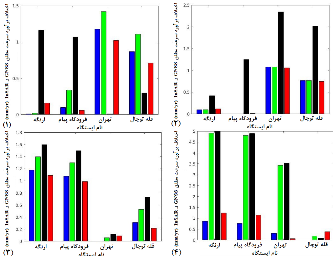
شکل ۱۰: اختلاف برآوردهای سرعت مطلق GNSS و InSAR نسبت به ایستگاه‌های ۱-ارنگه ۲- فرودگاه پیام ۳- تهران ۴- قله توچال. نمودارهای آبی، سبز، مشکی و قرمز به ترتیب نشان‌دهنده روش‌های اول تا چهارم هستند.
