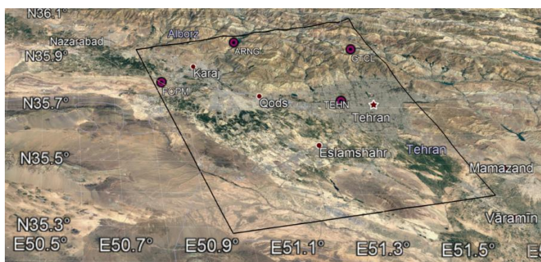
شکل ۳: منطقه مطالعاتی و ایستگاه‌های ژئودینامیک موجود در منطقه
