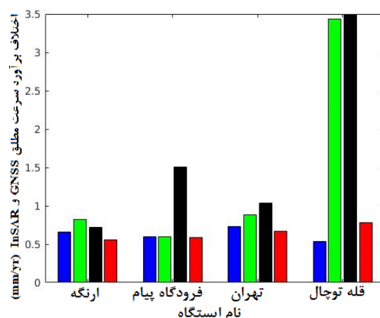
شکل ۱۱: خطای RMSE ایستگاه‌های ژئودینامیک. نمودارهای آبی، سبز، مشکی و قرمز به ترتیب نشان‌دهنده روش‌های اول تا چهارم هستند.
