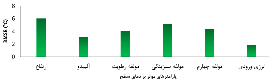
شکل ۷: RMSE بین مقادیر دمای سطح مدل شده و دمای سطح لندست ۸
