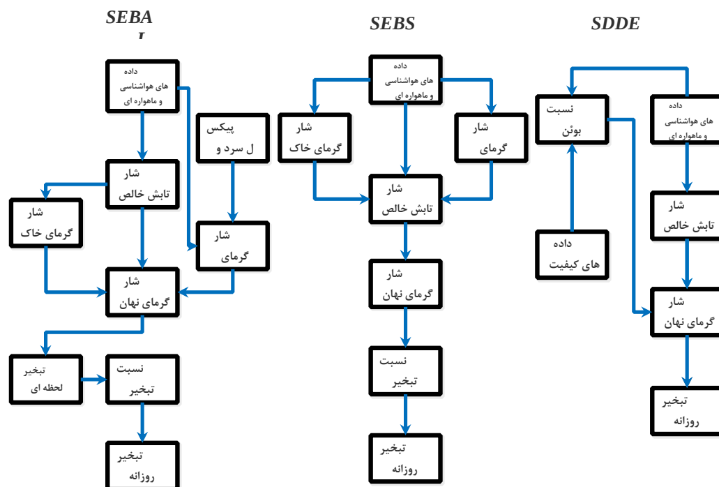
شکل ۲: خلاصه روش محاسباتی برآورد تبخیر با استفاده از سه مدل SEBS، SEBAL و SDD
