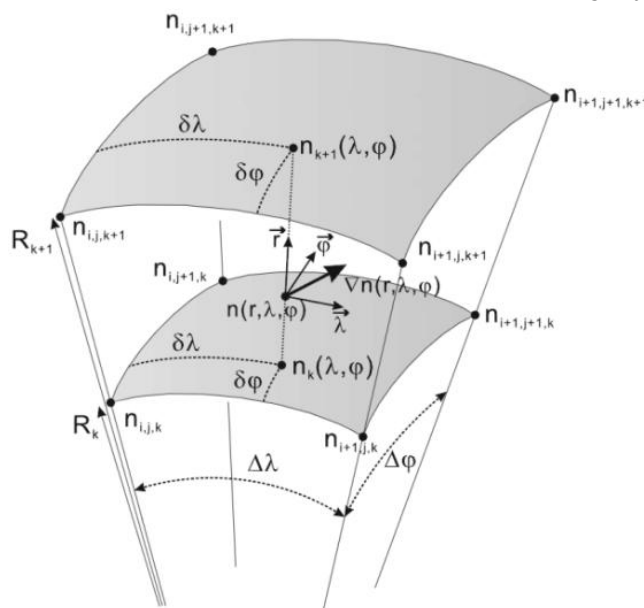
شکل ۲: ردیابی اشعه سه بعدی [۲]
