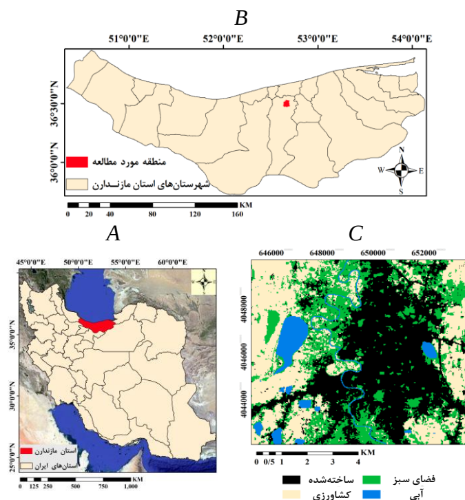
شکل ۲: منطقه مورد مطالعه (a) موقعیت جغرافیایی استان مازندران در ایران، (b) موقعیت جغرافیایی منطقه مورد مطالعه در استان مازندران و (c) کاربری های اراضی منطقه مورد مطالعه
