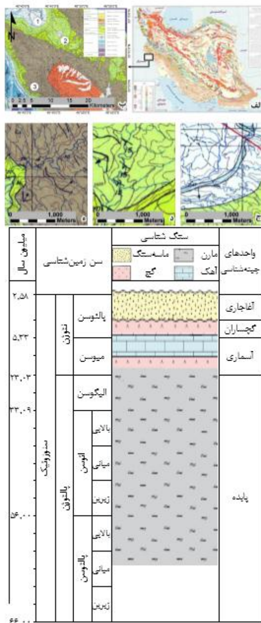
شکل ۳: منطقه و موقعیت سایت های مورد مطالعه بر روی نقشه زمین شناسی «ناران» (الف) منطقه مورد مطالعه در ایران؛ (ب) موقعیت سایت های مورد مطالعه بر روی نقشه زمین شناسی؛ (ج) سایت ۱ واقع بر روی سازند پایده-گورپی-صاف؛ (د) سایت ۲ واقع بر روی سازند آسماری-زیر و خشن؛ (ه) سایت ۳ بر روی سازند گچساران یا زیری متوسط؛ (و) نمودار چینه شناسی منطقه.
