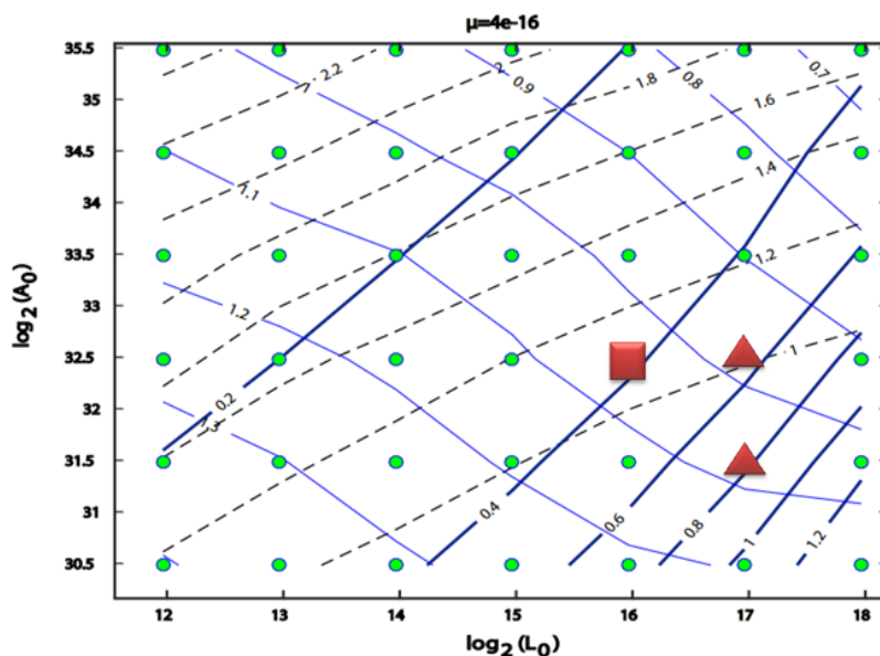
شکل ۴: مقادیر معیار خطا در مدل‌های با \mu = 4 \times 10^{-16} \text{ s}^{-1} و A_0, L_0 متغیر. خطوط نازک، ضخیم و خطچین به ترتیب معرف معیارهای N_2^{\text{sterr}} ، N_2^{\text{potency}} ، N_2^{\text{geodetic}} می‌باشند مدل‌های قابل قبول و انتخاب شده به ترتیب به صورت مثلث و مربع نشان داده شده است.
