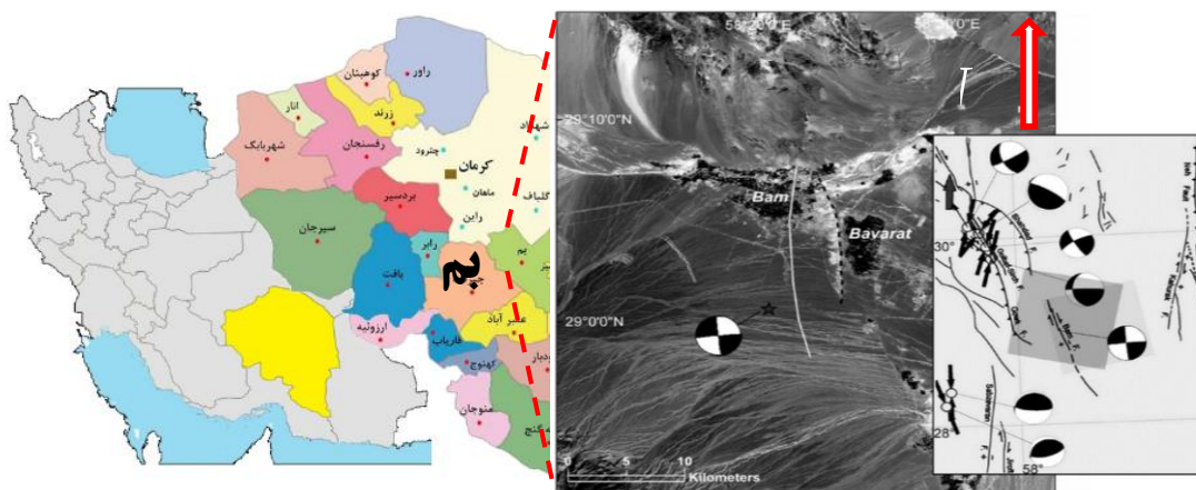
شکل ۱: موقعیت بم و بروات در کرمان، موقعیت گسل بم و انشعابات آن و سازوکار کانونی زلزله ۱۳۸۲ بم [۵۱]
