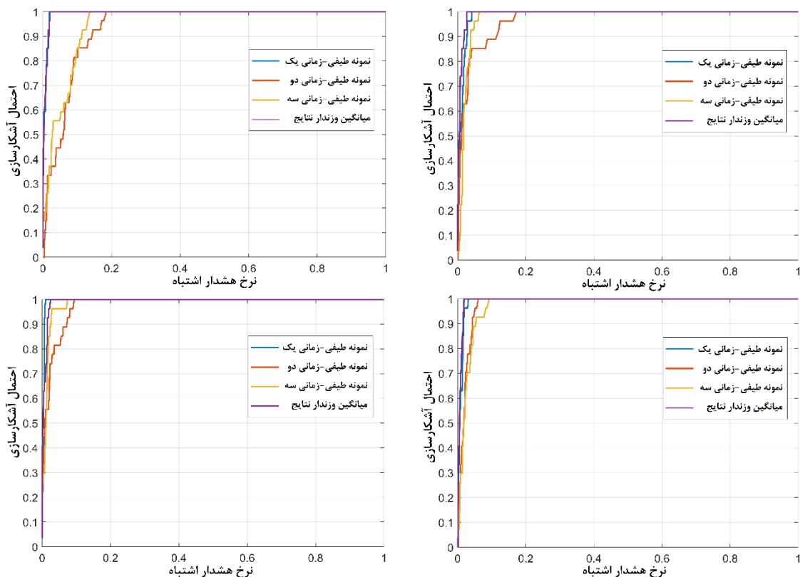
شکل ۷: نمودار ROC مربوط به بهینه سازی برای سه طیف انتخابی و میانگین نتایج برای روش های آشکارسازی معرفی شده؛ (الف) CEM (ب) ACE (پ) MF (ت) ASMF
