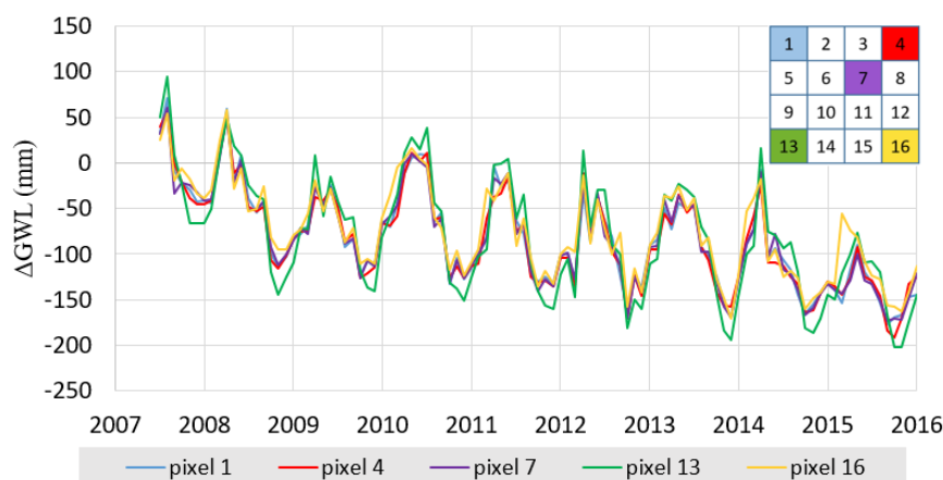
شکل ۹: سری های زمانی ریزمقیاس شده مربوط به تغییرات سطح آب های زیرزمینی با مقیاس ۰٫۲۵°، سری زمانی مربوط به هر پیکسل با رنگ متناظر آن نشان داده شده است.
