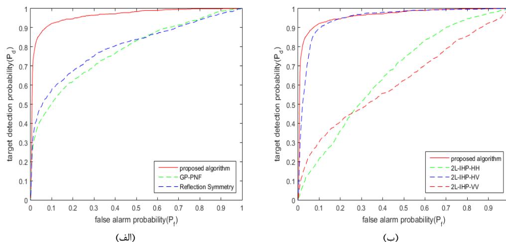
شکل ۹: منحنی ROC مربوط به (الف) روش پیشنهادی و GP-PNF و (ب) روش پیشنهادی و 2L-IHP در کانال‌های HH و VV و HV
