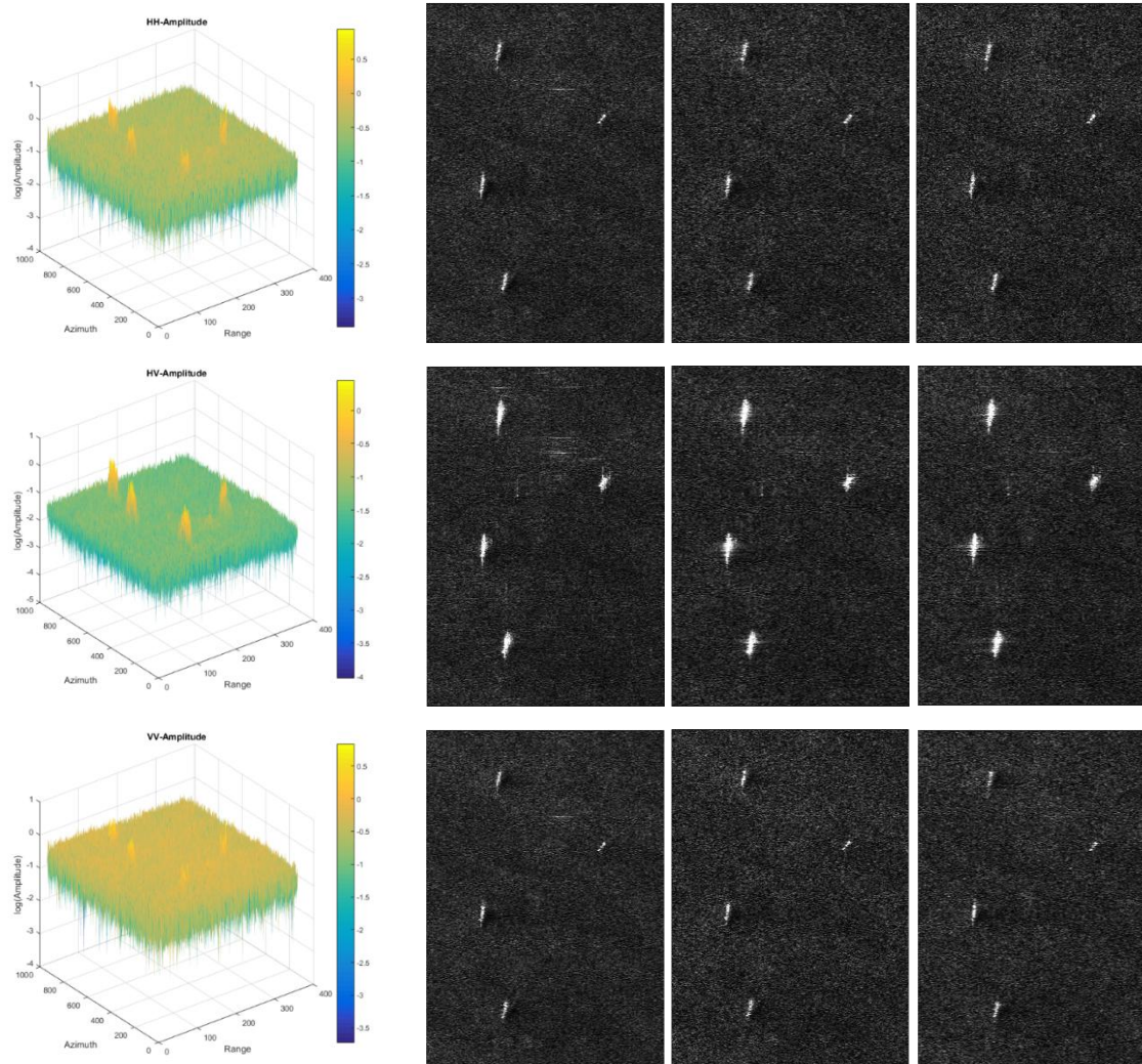
شکل ۵: سطر اول از بالا مربوط به کانال HH ، سطر دوم مربوط به کانال HV و سطر سوم مربوط به کانال VV است. و ستون اول، دوم و سوم و چهارم از چپ به راست به ترتیب نمودار سه بعدی، تصاویر دامنه، زیرمنظر اول و زیرمنظر دوم را نشان می‌دهند. تمامی این تصاویر مربوط به پایه پلاریزاسیون با پارامترهای هندسی بیضی \tau = \varphi = 0 می‌باشد.
