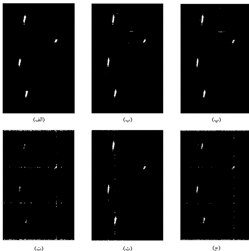
شکل ۸: نتایج آشکارسازی کشتی برای تصویر نشان داده شده در شکل ۵ با استفاده از (الف) روش پیشنهادی \Lambda_N ، (ب) GP- \Lambda_N ، (پ) روش تقارن بازتابی، (ت) 2L-IHP در کانال HH، (ث) 2L-IHP در کانال HV، (ج) 2L-IHP در کانال VV.
