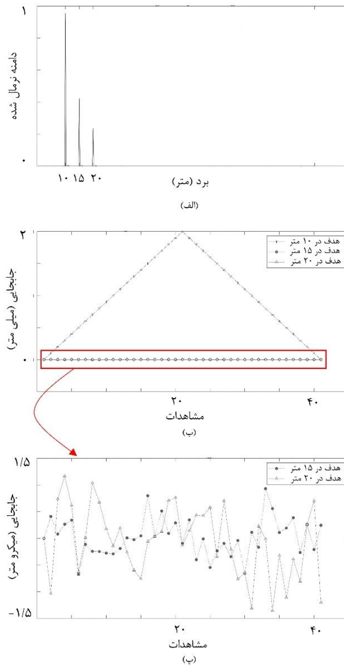
شکل ۷: شبیه‌سازی پایش جایبایی در حالت رادار با حضور سه هدف. (الف) سیگنال فشرده‌شده (ب) جایبایی اهداف در پایش سری زمانی (پ) بررسی خطای جایبایی مشاهده‌شده در طول پایش برای دو هدف ثابت
