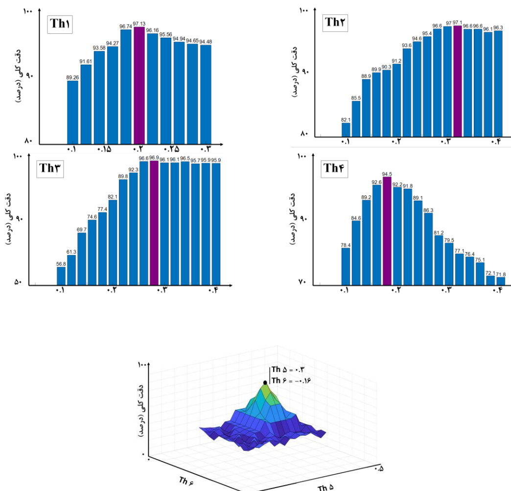
شکل ۸: مقادیر دقت به‌ازای حد آستانه‌های مختلف (جست و جوی شبکه‌ای)
