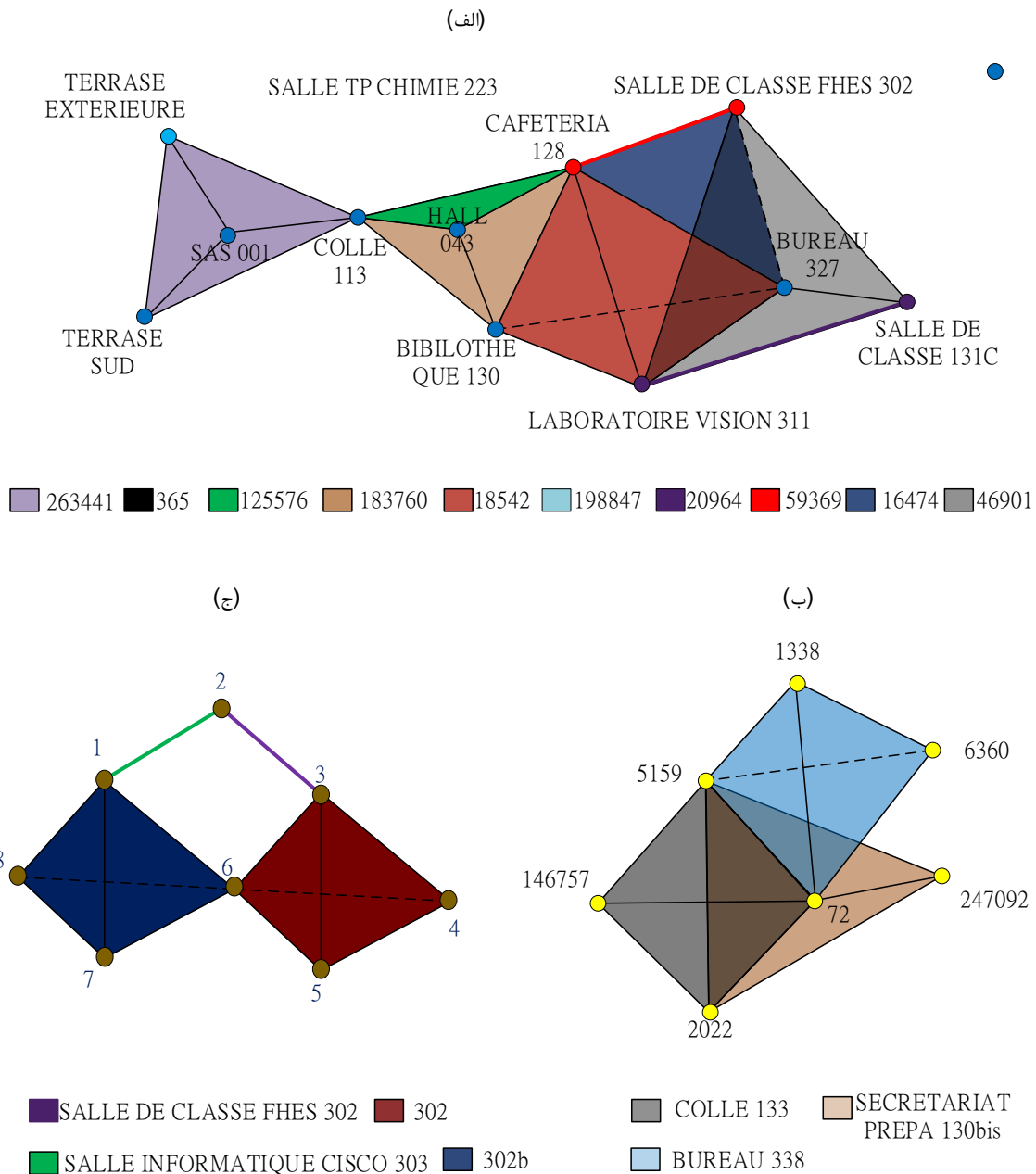
شکل ۴: تعبیر هندسی سه مجتمع سادگی نمونه
