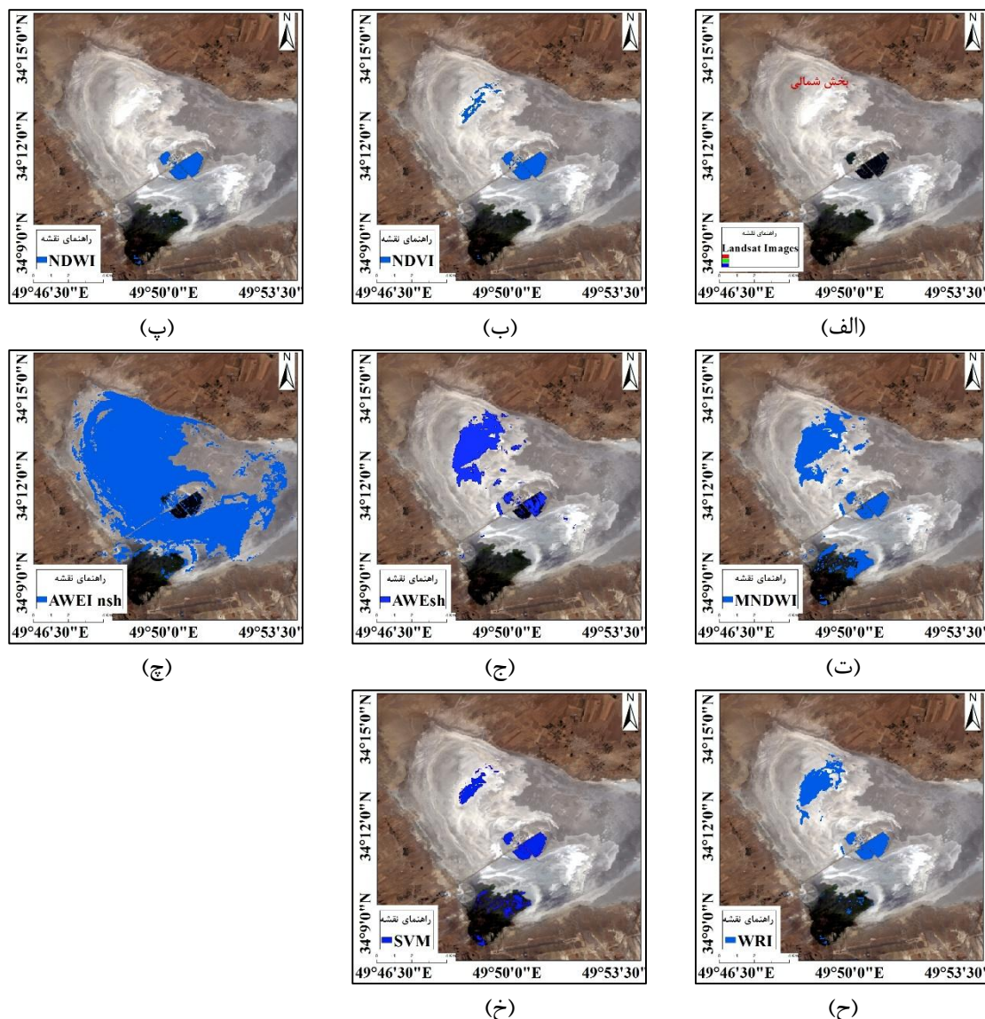
شکل ۴: مقایسه نتایج اعمال شاخص های مختلف در استخراج پهنه آبی تالاب در وضعیت کم آبی: (الف) تصویر لندست ۸ ترکیب رنگی باند ۴-۳-۲ در تاریخ: ۲۰۱۴/۰۷/۰۸، (ب) شاخص NDVI، (پ) شاخص NDWI، (ت) شاخص MNDWI، (ج) شاخص AWEI sh ، (چ) شاخص AWEI nsh ، (ح) شاخص WRI، (خ) طبقه بندی SVM
