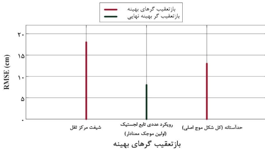
شکل ۱۷: نمودار میله‌ای معرفی نتایج عددی ارزیابی سری زمانی ارتفاع آب حاصل از رویکردهای بهینه مختلف باز تعقیب در مقایسه با داده‌های نوسان نگار محلی
