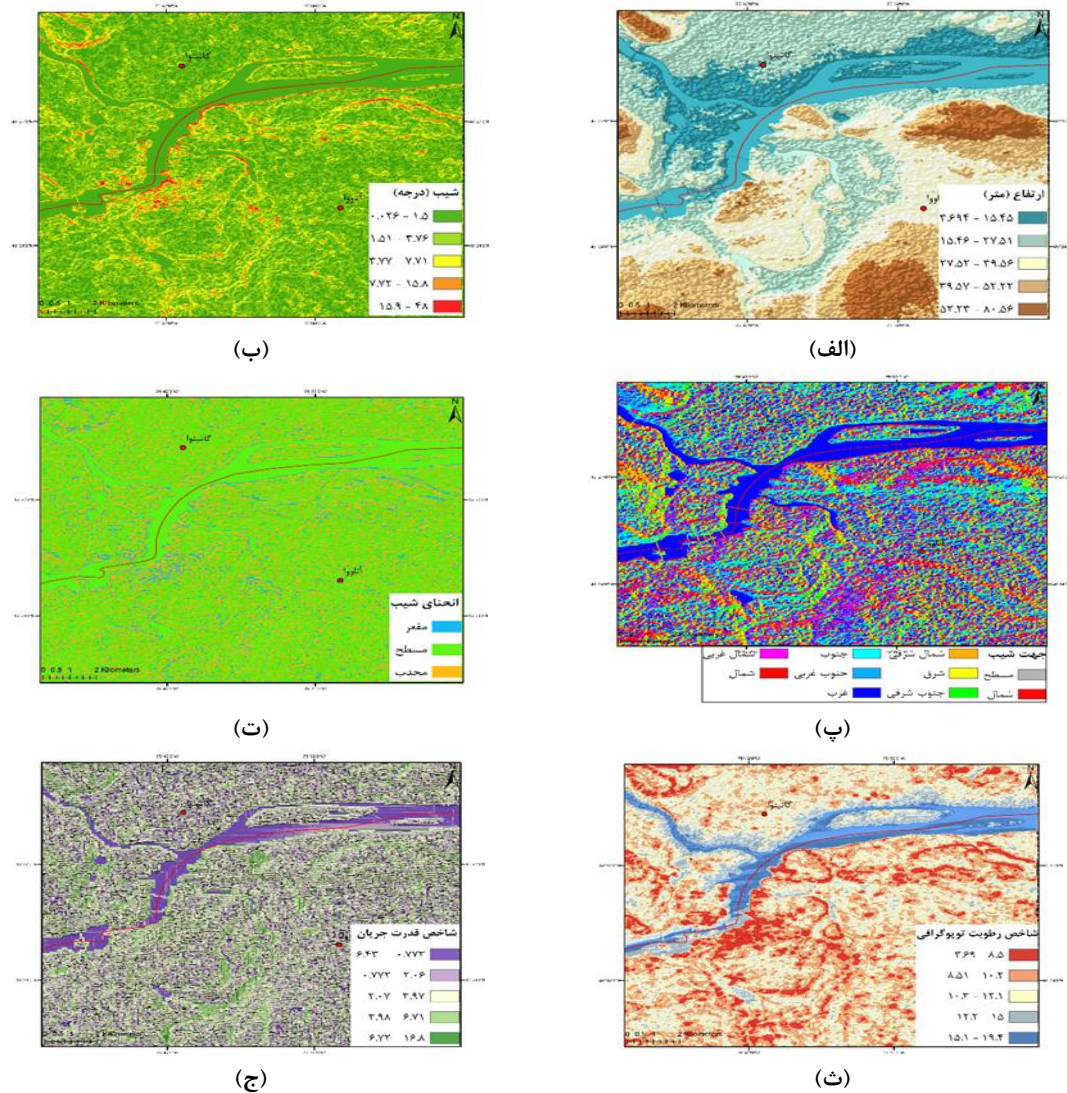
شکل ۱۳: نقشه مستخرج از DEM تولید شده از تصاویر TerraSar-x، نقشه ارتفاع، (ب) نقشه شیب، (پ) نقشه جهت شیب، (ت) نقشه انحنای شیب، (ث) نقشه شاخص TWI، (ج) نقشه شاخص SPI
