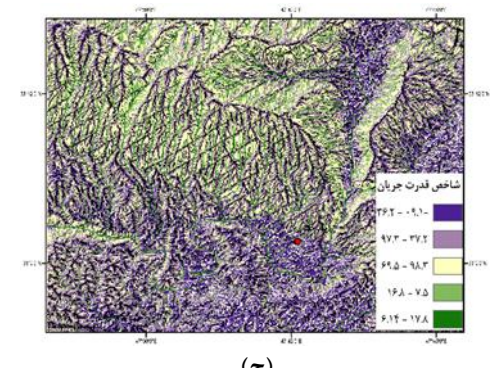
شکل ۱۶: نقشه متغیرهای سنجش از دوری، (الف) نقشه شاخص پوشش گیاهی، (ب) نقشه کاربری اراضی، (پ) نقشه ارتفاع، (ت) نقشه شیب، (ث) نقشه جهت شیب، (ج) نقشه انحنای شیب، (چ) نقشه TWI ، (ح) نقشه SPI
