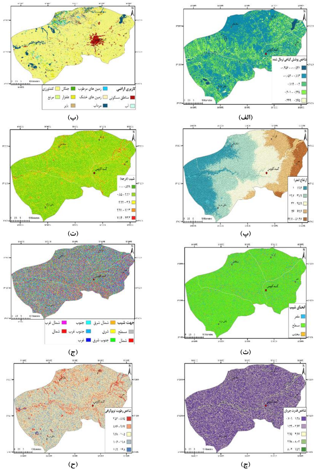
شکل ۷: نقشه متغیرهای سنجش از دوری منطقه گندکاووس، (الف) نقشه پوشش گیاهی، (ب) نقشه کاربری اراضی، (پ) نقشه ارتفاع، (ت) نقشه شیب، (ث) نقشه جهت شیب، (ج) نقشه انحنای شیب، (ح) نقشه شاخص رطوبت توپوگرافی، (ح) نقشه شاخص قدرت جریان
