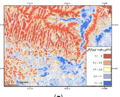
شکل ۱۶: نقشه متغیرهای سنجش از دوری، (الف) نقشه شاخص پوشش گیاهی، (ب) نقشه کاربری اراضی، (پ) نقشه ارتفاع، (ت) نقشه شیب، (ث) نقشه جهت شیب، (ج) نقشه انحنای شیب، (چ) نقشه TWI ، (ح) نقشه SPI
