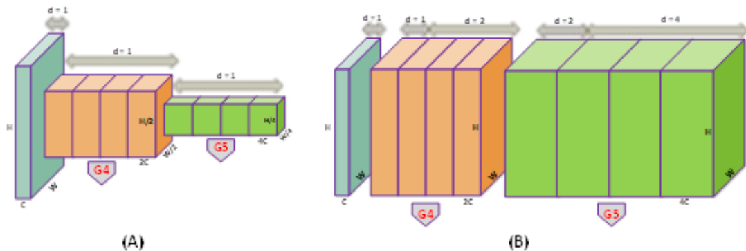
شکل ۳: مقایسه اصلی ResNet (ستون A) با ResNet گسترده (ستون B). در اینجا، H و C به ترتیب ارتفاع، عرض و تعداد کانال‌های یک نقشه ویژگی میانی را نشان می‌دهند. d=1 نشان دهنده یک کانولوشن استاندارد است. سایر مقادیر d نشان‌دهنده نرخ‌های مختلف مورد استفاده در کانولوشن است.
