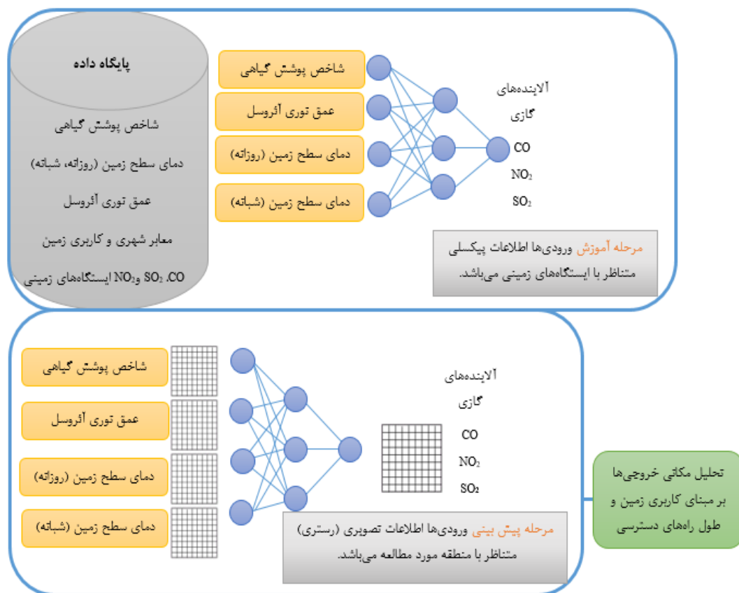
شکل ۱: مدل مفهومی روش پیشنهادی
