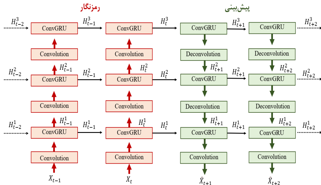
شکل ۱: ساختار رمزگذار-پیش‌بینی کننده به کار گرفته شده در مدل پیشنهادی برای پیش‌بینی درختش‌های یونسفری
