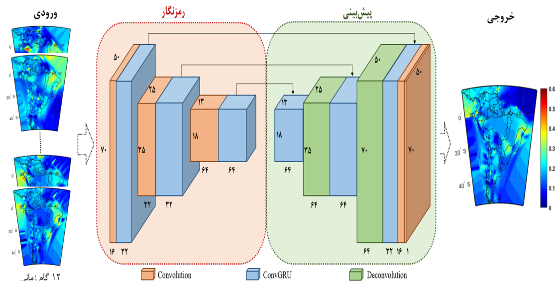
شکل ۲: ساختار مدل مبتنی بر روش ConvGRU برای پیش‌بینی منطقه‌ای درخشش‌های یونسفری در منطقه آمریکای جنوبی
