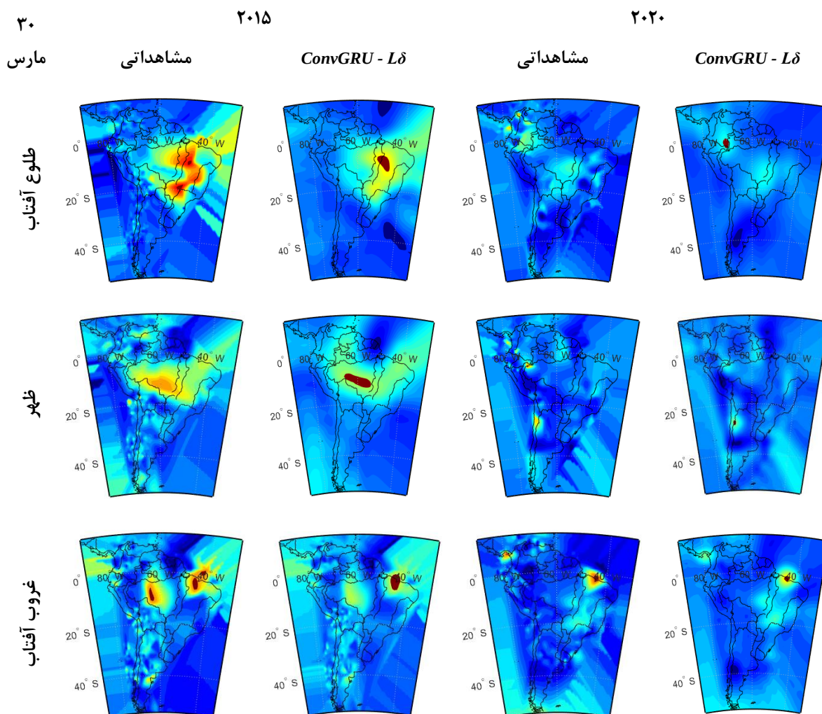
شکل ۶: مقادیر S4 مشاهداتی و پیش‌بینی‌شده برای محدوده آمریکای جنوبی در روز ۳۰ام مارس در سه بازه زمانی هنگام طلوع خورشید (Sunrise)، هنگام ظهر (Noon) و هنگام غروب آفتاب (Sunset). ستون اول و دوم به ترتیب مقادیر مشاهداتی و پیش‌بینی‌شده S4 برای سال ۲۰۱۵ و ستون‌های سوم و چهارم مقادیر ترتیب مقادیر مشاهداتی و پیش‌بینی‌شده S4 برای سال ۲۰۲۰
