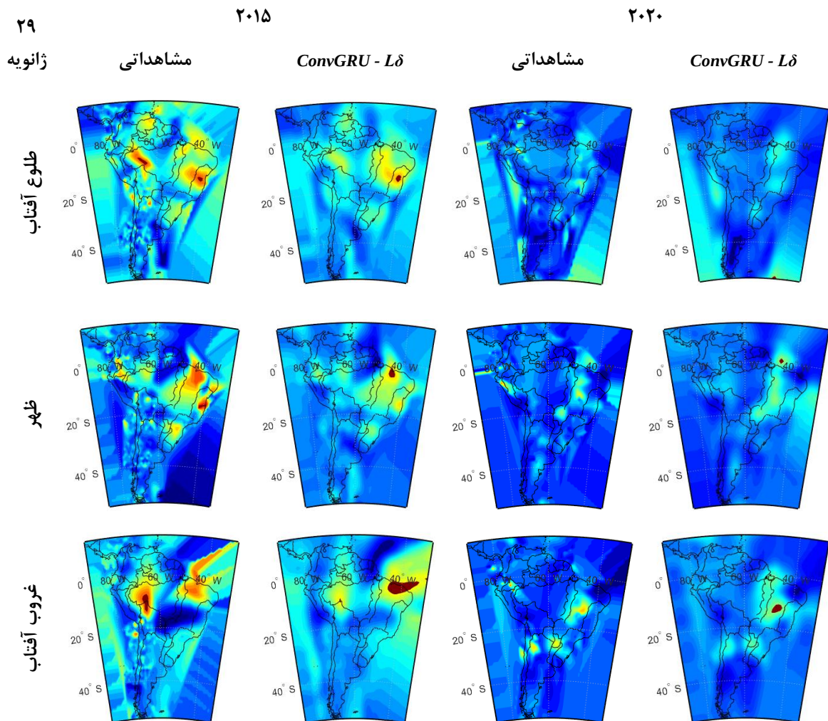
شکل ۵: مقادیر S4 مشاهداتی و پیش‌بینی شده برای محدوده آمریکای جنوبی در روز ۱۲م ژانویه در سه بازه زمانی هنگام طلوع خورشید (Sunrise)، هنگام ظهر (Noon) و هنگام غروب آفتاب (Sunset). ستون اول و دوم به ترتیب مقادیر مشاهداتی و پیش‌بینی شده S4 برای سال ۲۰۱۵ و ستون‌های سوم و چهارم مقادیر ترتیب مقادیر مشاهداتی و پیش‌بینی شده S4 برای سال ۲۰۲۰
