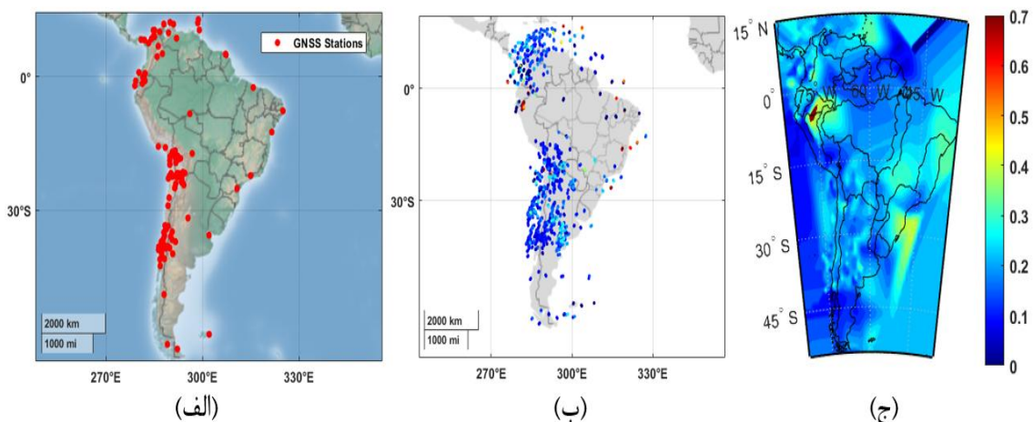
شکل ۳: (الف) توزیع جغرافیایی ایستگاه‌های GNSS در محدوده آمریکای جنوبی، (ب) مشاهدات S4 در امتداد مسیر IPP در ساعت (UT) ۱۴:۰۰ در ۱۵ ژانویه ۲۰۱۵ و (ج) یک نمونه نقشه S4 که از طریق درون‌یابی با استفاده از روش کریجینگ
