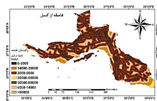
۴-۱۵- نقشه فاصله از گسل
