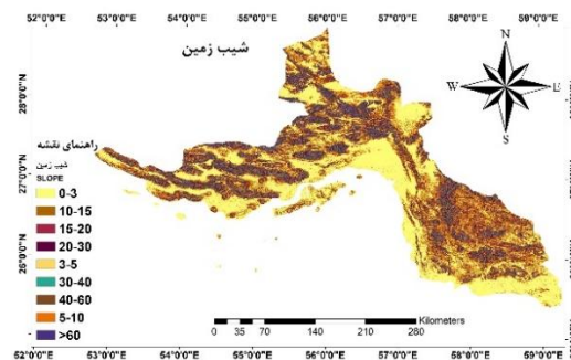
۴-۲۲- نقشه شیب زمین
