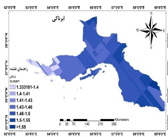
۴-۱- نقشه ابرناکی
