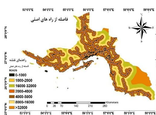
۴-۱۳- نقشه فاصله از راه‌های اصلی
