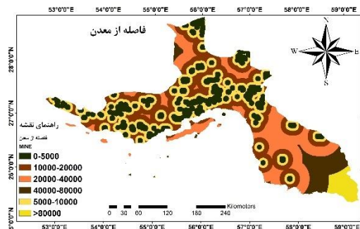
۴-۲۱- نقشه فاصله از معدن
