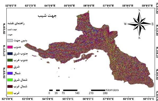
۴-۱۹- نقشه جهت شیب
