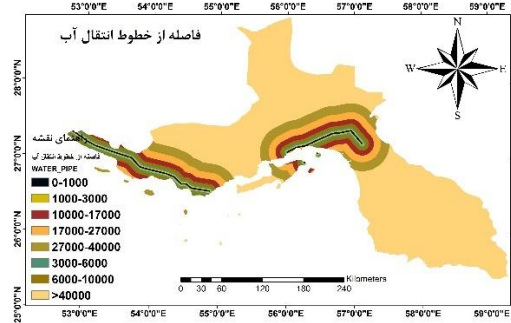
۴-۱۷- نقشه فاصله از خطوط انتقال آب
