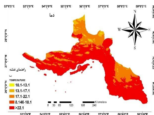
۴-۱۰- نقشه دما
