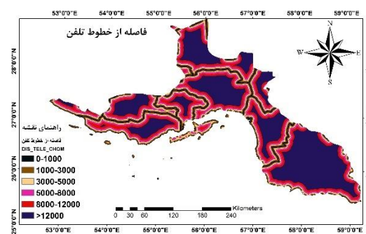
۴-۱۶- نقشه فاصله از خطوط تلفن
