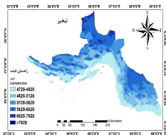
۴-۲- نقشه تبخیر
