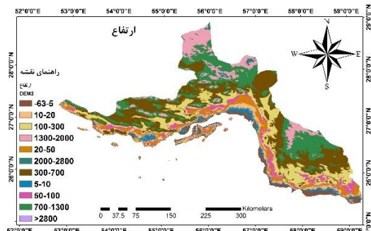
۴-۲۳- نقشه ارتفاع
