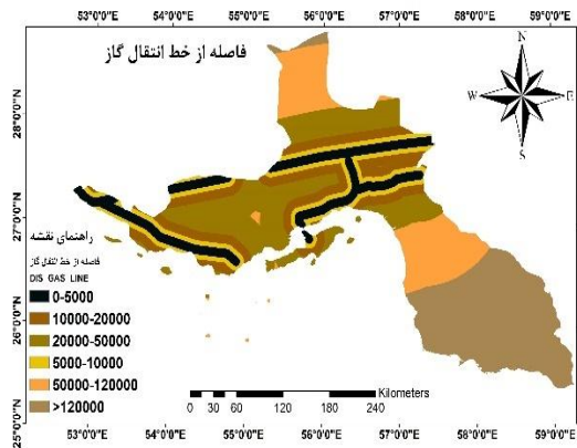
۴-۱۲- نقشه فاصله از خط انتقال گاز
