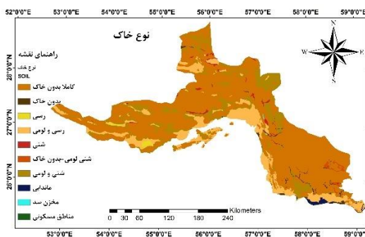
۴-۲۰- نقشه نوع خاک
