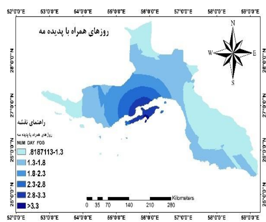
۴-۵- نقشه روزهای همراه با پدیده مه
