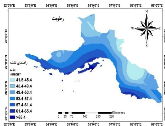
۴-۷- نقشه رطوبت
