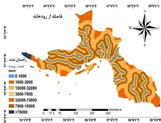
۴-۱۴- نقشه فاصله از رودخانه
