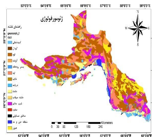
۴-۲۶- نقشه ژئومورفولوژی
