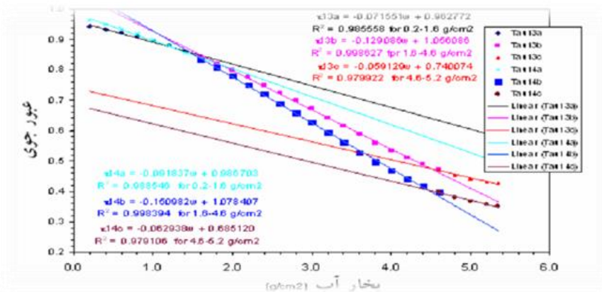
شکل ۱: نمودار میزان قابلیت عبور جو برای مقادیر مختلف بخار آب جو
