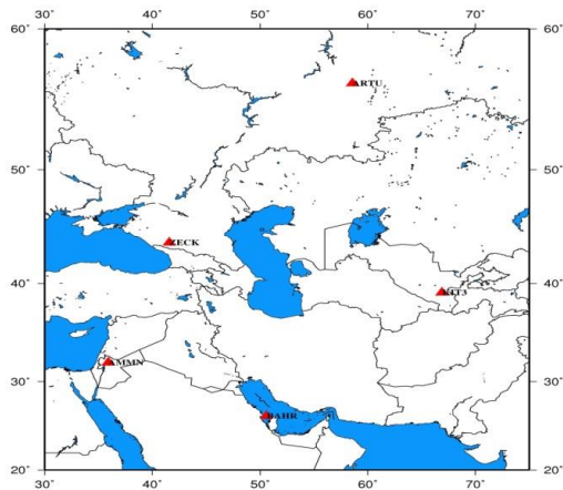
شکل ۲. ایستگاه‌های GNSS مورد استفاده در پردازش داده‌های این تحقیق. محل ایستگاه‌های مورد استفاده از این شبکه با مثلث نشان داده شده، و نام اختصاری هر ایستگاه در کنار محل هر ایستگاه به نمایش درآمده است.
