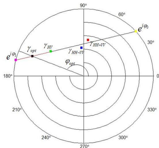
شکل ۳: نمایش موقعیت همدوسی حجمی بهینه بر روی خط همدوسی در مقایسه با همدوسی حجمی مورد استفاده در روش مرسوم سه‌مرحله‌ای در داده QP . مقادیر همدوسی در پایه‌های پائولی به ترتیب با رنگ‌های آبی، قرمز و سبز نشان داده شده‌است. همدوسی زمینی با نام e^{i\phi_0} و با رنگ زرد نمایش داده شده‌است. همدوسی حجمی بهینه حاصل از روش ESPO با رنگ مشکی و با عنوان \gamma_{opt} دیده می‌شود [۱۲].
