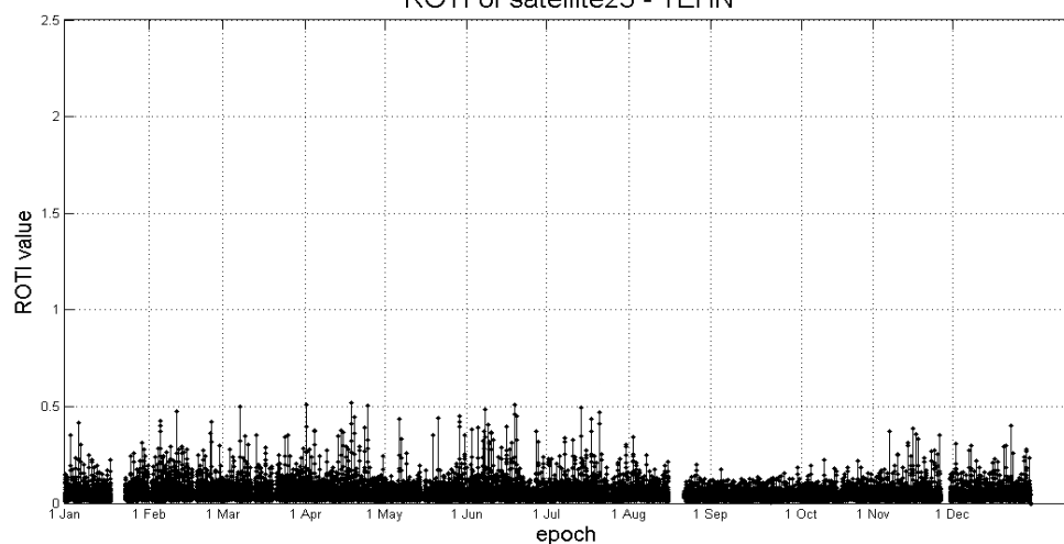
شکل ۳: ROTI استخراج شده برای ایستگاه تهران در سال ۲۰۱۵ و ماهواره شماره ۲۳
