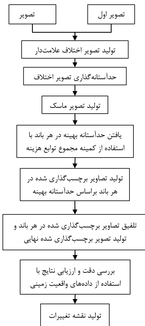
شکل ۲: فلوچارت روش پیشنهادی
