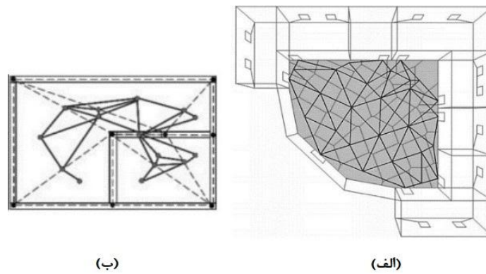
شکل ۲: تولید شبکه ناوبری در فضای داخلی ساختمان: (الف) با استفاده از دیاگرام ورونویی [۱۷]، (ب) با استفاده از مثلث‌بندی نامنظم [۱۵]
