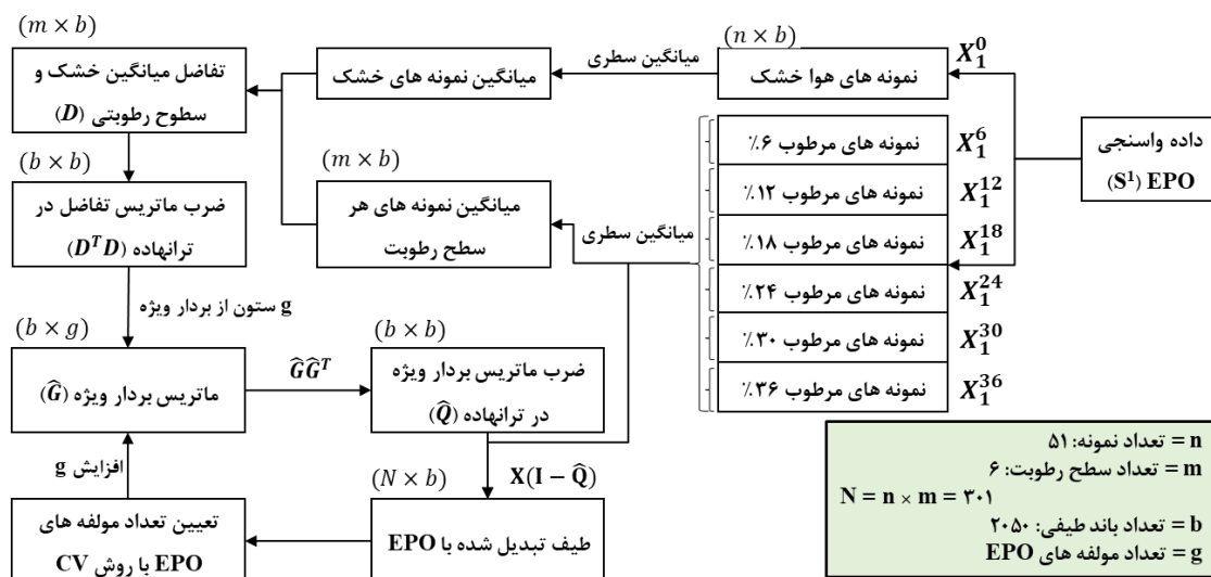
شکل ۳: نحوه پیاده‌سازی الگوریتم EPO برای پارمتر رطوبت.
