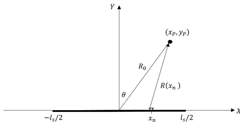
شکل ۴: هندسه تصویربرداری روزنه مصنوعی در سیستم رادار زمینی
