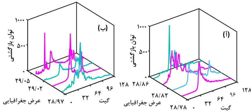
شکل ۲: نمونه شکل موج‌های منطقه مطالعاتی (آ) گذر ۱۳۹، دوره ۴۰ و (ب) گذر ۲۵، دوره ۲۰
