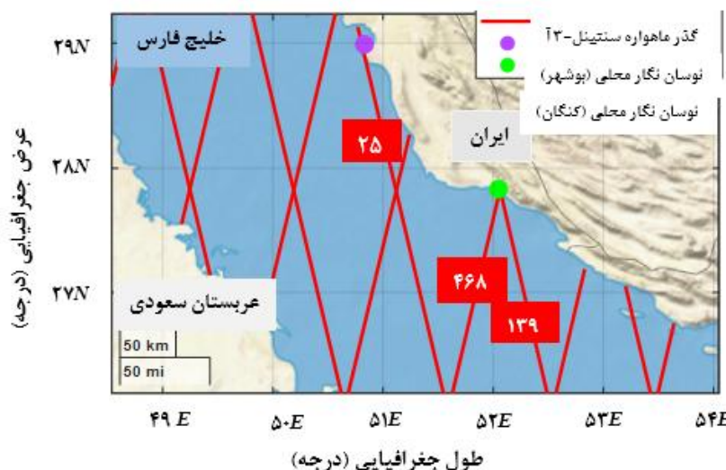
شکل ۱: موقعیت گذرهای انتخابی مأموریت سنتینل-۳ و نوسان‌نگارهای محلی در منطقه ساحلی خلیج فارس
