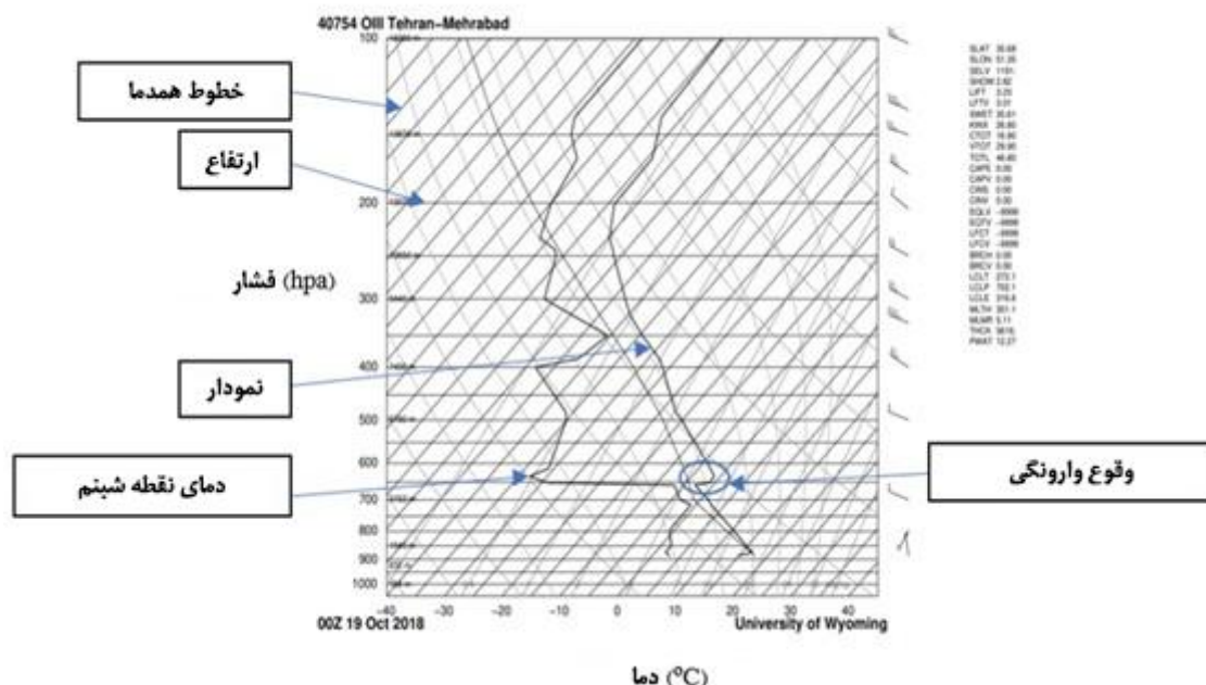
شکل ۲: نمایش نمونه‌ای از یک نمودار skew-T [۲۱]
