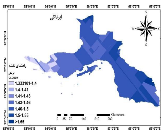
۱-۴- نقشه ابرناکی
