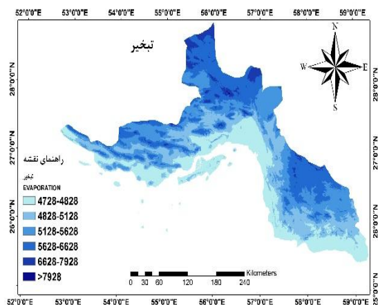
۲-۴- نقشه تبخیر
