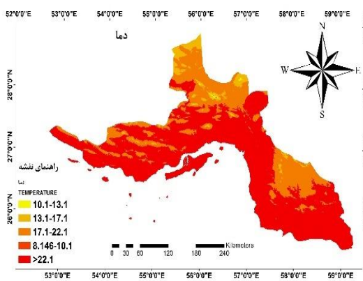
۴-۱۰- نقشه دما
