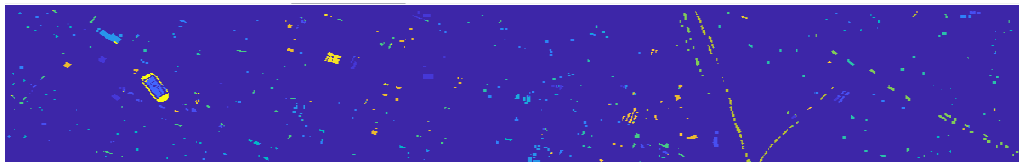
MMP-CNN
