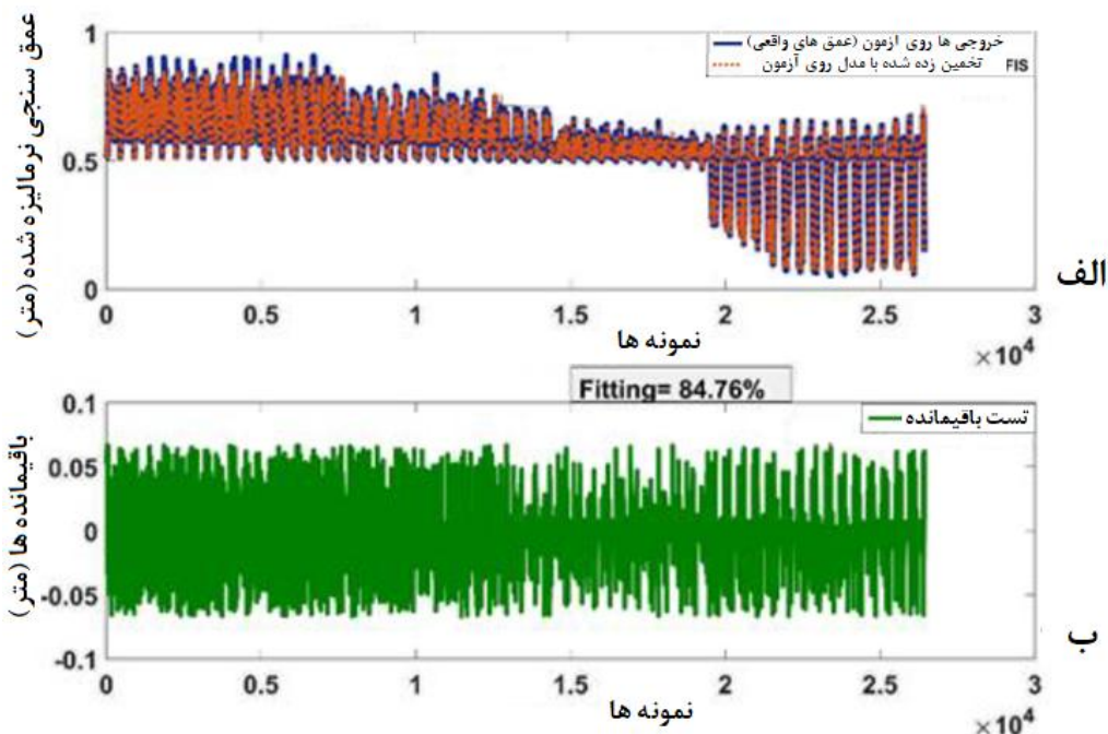
شکل ۵: مدل‌سازی عمق سنجی با استفاده از ANFIS روی داده‌های آزمون شامل (الف) عمق نرمالیزه شده و (ب) باقیمانده‌های بین داده‌های واقعی و برآورد شده با مدل
