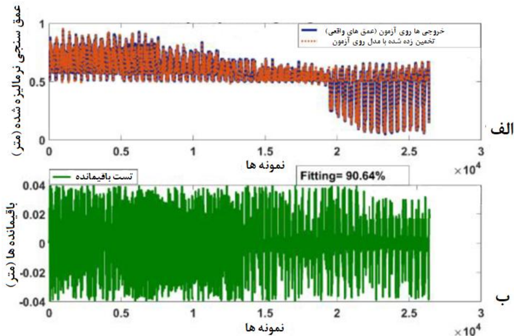
شکل ۶: مدل سازی عمق سنجی با استفاده از LOLIMOT روی داده های آزمون شامل (الف) عمق نرمالیزه شده و (ب) باقیمانده های بین عمق حاصل از داده های واقعی و برآورد شده با مدل
