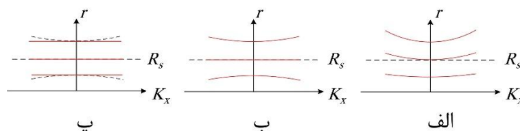
شکل ۲: تاثیر اعمال فیلتر منطبق و تبدیل استولت در برطرف کردن انحنای برد اهداف در الگوریتم RMA: الف) سیگنال فشرده-شده در برد قبل از تصحیح انحنای برد اهداف نسبت به خط برد مرجع با اعمال فیلتر منطبق دوبعدی (رابطه (۱۲)). ب) تصحیح انحنای برد اهداف پس از تبدیل و درون‌یابی استولت
