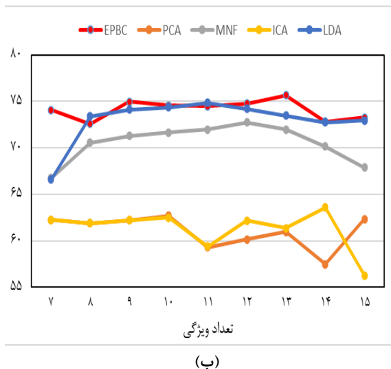
شکل ۴: نمودار دقت کلی طبقه بندی برای تصویر کاج‌های هندی، الف: ۱۰٪ نمونه آموزشی، ب: ۲۰٪ نمونه آموزشی
