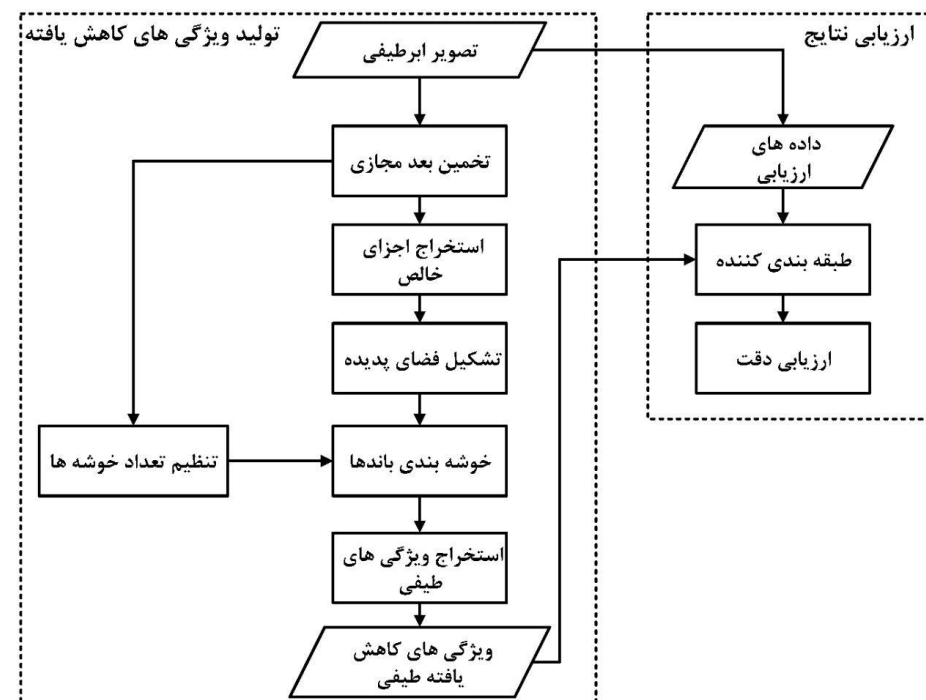
شکل ۱: فلوچارت روش پیشنهادی (EPBC)
